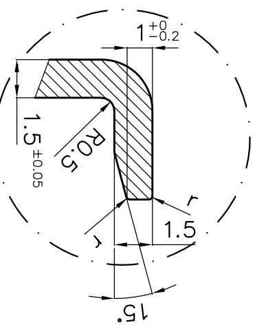
DETTAGLIO X
